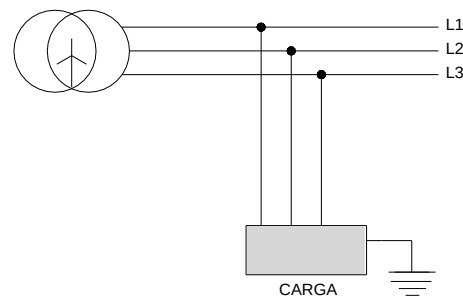
Figura 5 - Esquema IT
