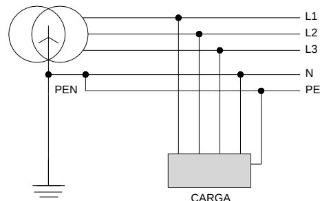
Figura 2 - Esquema TN-C-S
